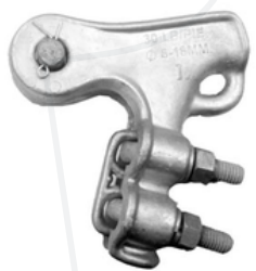
✓ GRAPA DE ANCLAJE TIPO PISTOLA - 2P (AL -AG)
